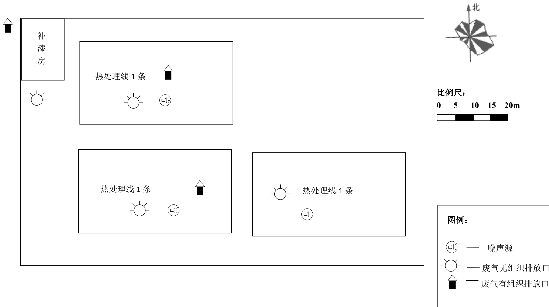
附图 3 生产车间 1 平面布置图
